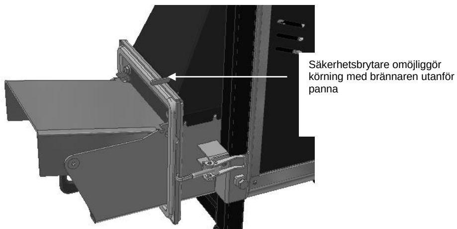
Figur 2 Säkerhetsbrytare
